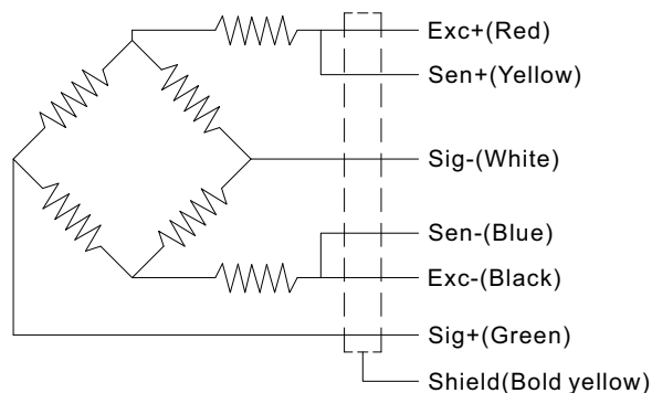
Wiring Code@Clockwise
